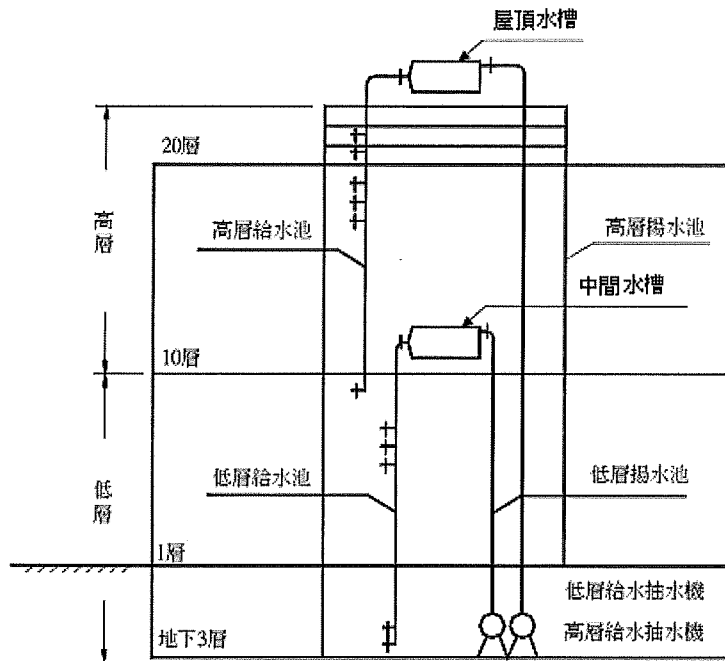
圖3-6 間接給水設置中間水槽示意圖
