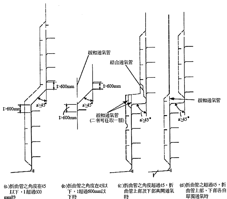
圖4-2 立管、折曲管與排水橫主管之關係
