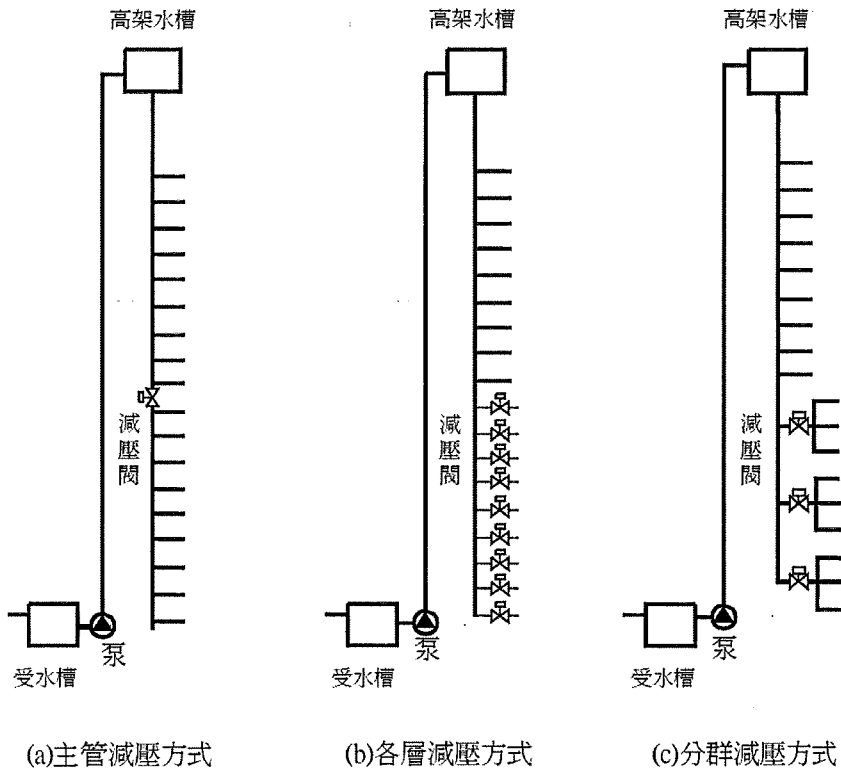
圖3-9 利用減壓閥之給水配管分區示意圖
