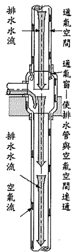
圖4-7 排水通氣二層管方式
