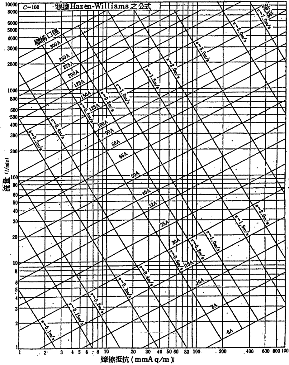
圖 A-5 配管用碳鋼鋼管摩擦抵抗線圖
