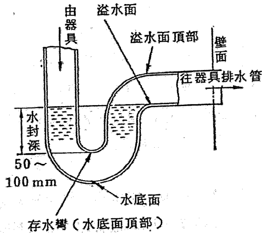
圖4-18 存水彎裝置封水深度圖例
