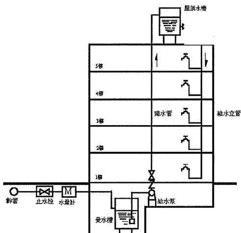
圖3-3 重力給水系統圖
