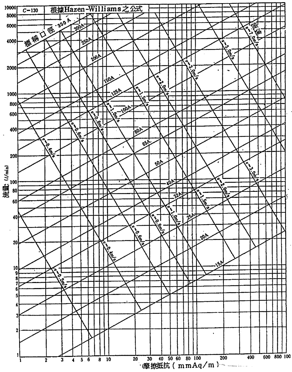
圖 A-7 內襯 PVC 鋼管摩擦抵抗線圖
