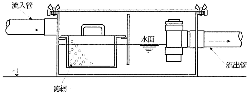
圖4-23 固體物截留器參考圖例
