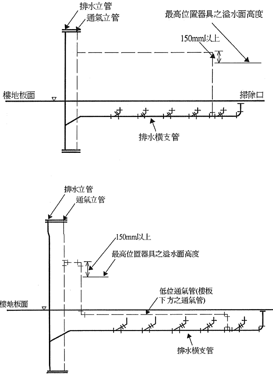
圖4-9 有條件之低位通氣管安裝圖例
