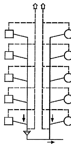
b. 全通氣二立管方式
