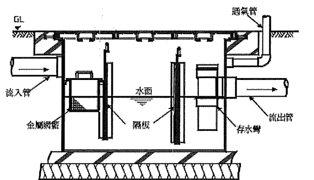
(a)工廠製造的截留器
