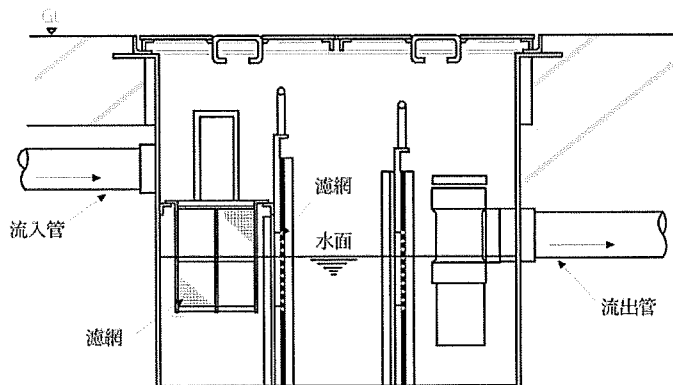
圖4-22 纖維毛髮截留器參考圖例
