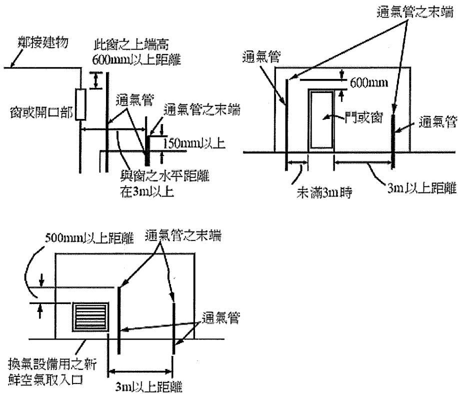
圖4-12 通氣管末端開口部之位置
