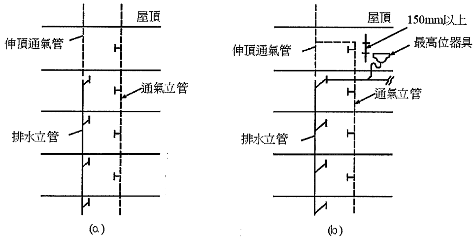
圖4-11 通氣立管上部處理
