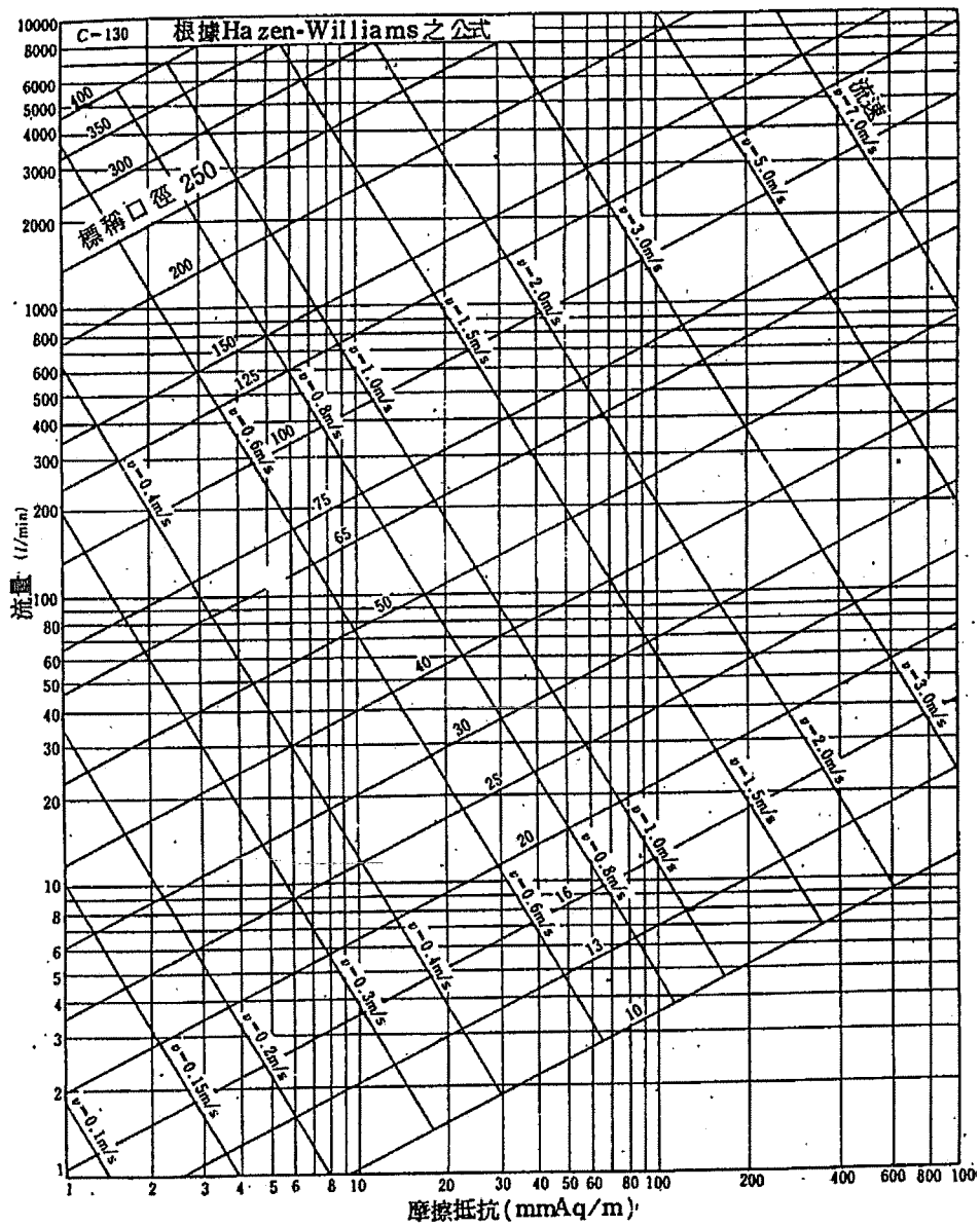
圖 A-6 PVC 管摩擦抵抗線圖
