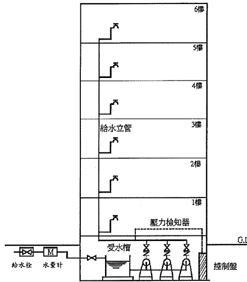
圖3-4 加壓泵給水系統圖
