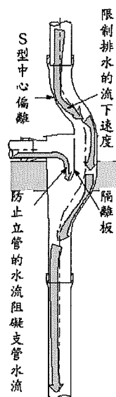
圖4-6 抑制排水流下速度方式
