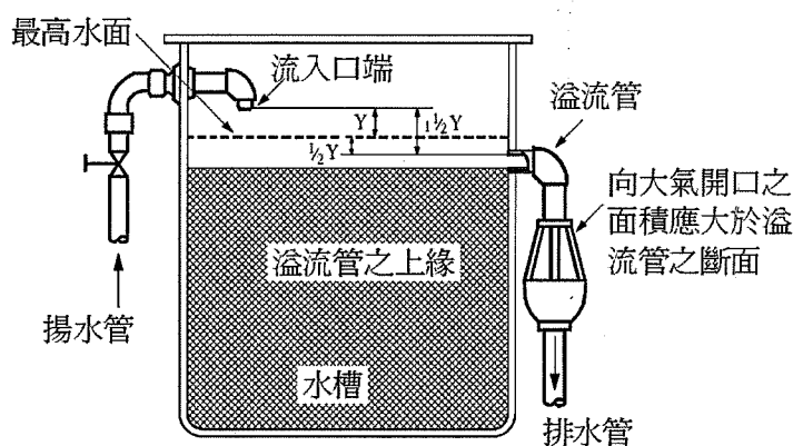
圖3-11 飲用水槽之出水口空間(B)
