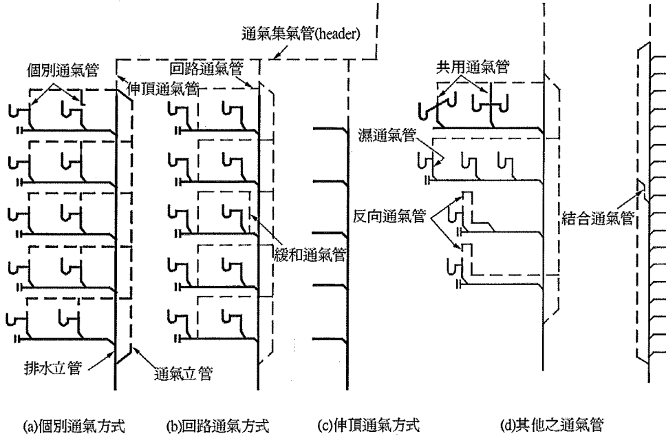
圖4-4 通氣方式與通氣管
