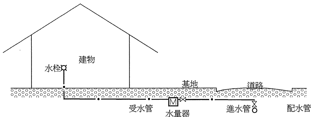
圖3-1 直接給水系統圖
