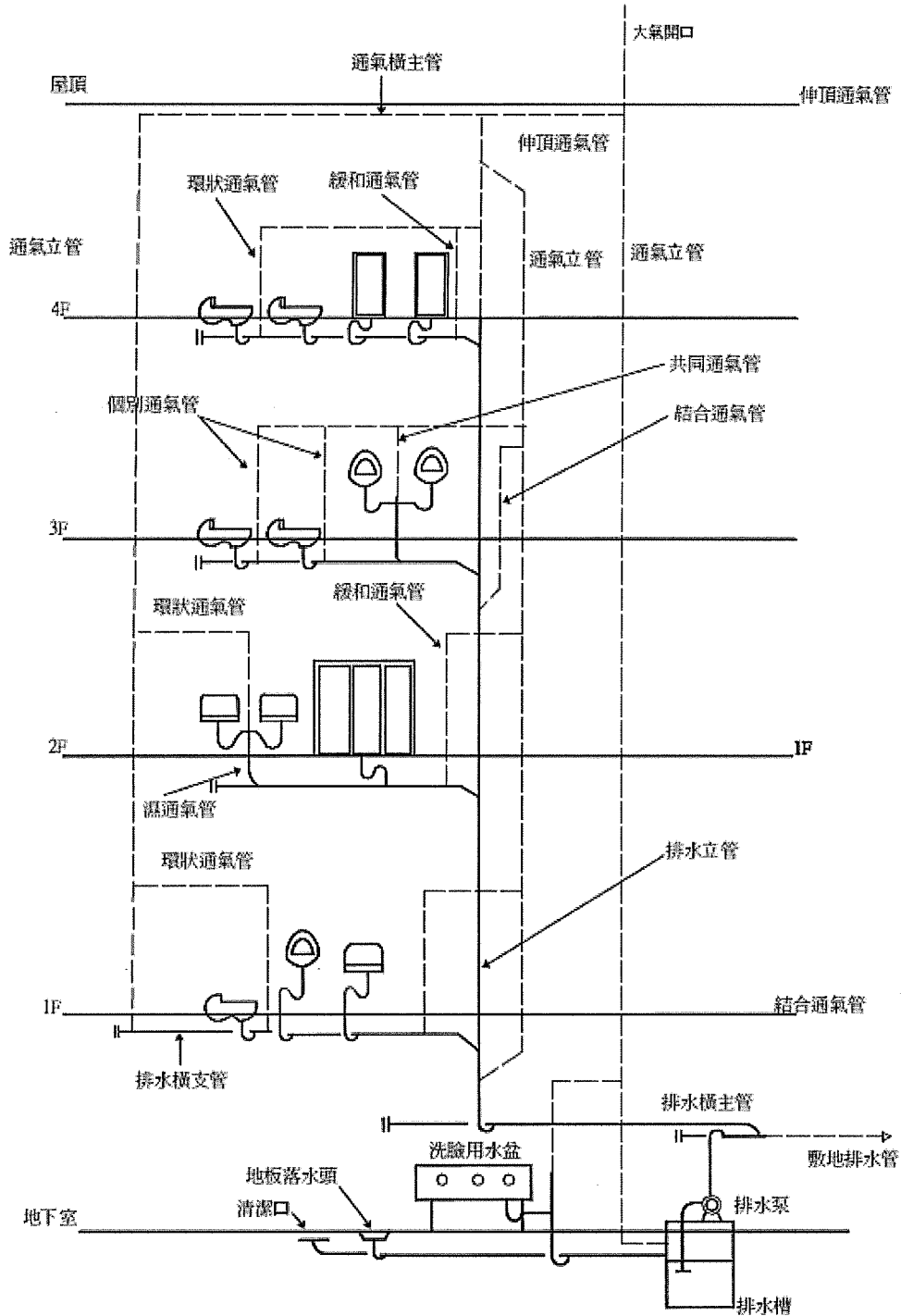
圖4-8 排水通氣系統圖
