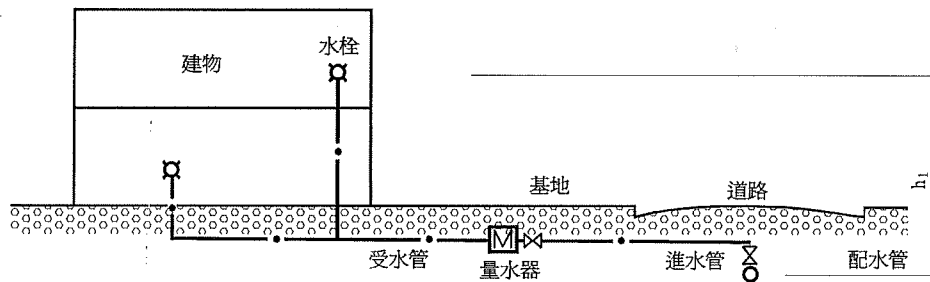
圖 A-3 自來水引入配管圖
