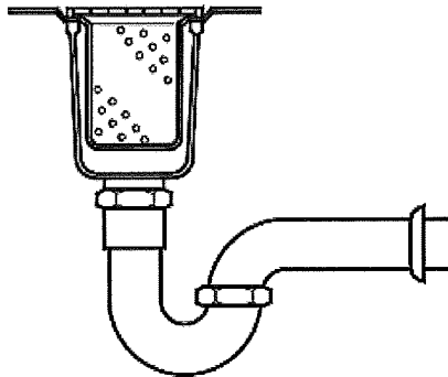
圖4-21 毛髮截留器參考圖例
