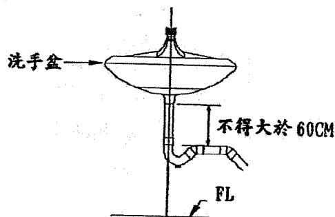
圖4-17 壁掛式洗手臺之存水彎設置
