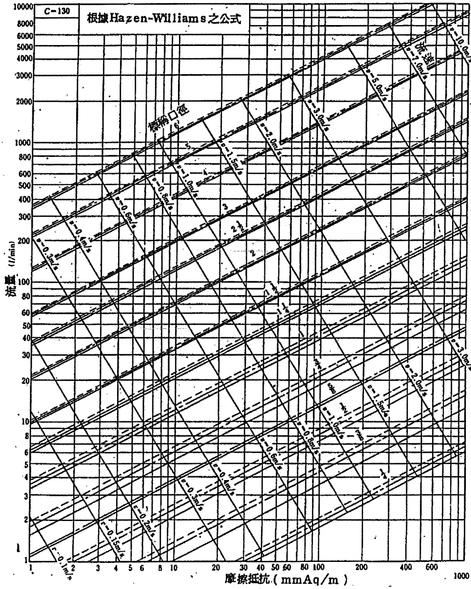
圖 A-8 銅管摩擦抵抗線圖
